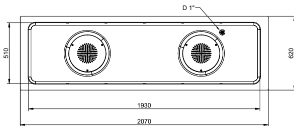
Päältä
